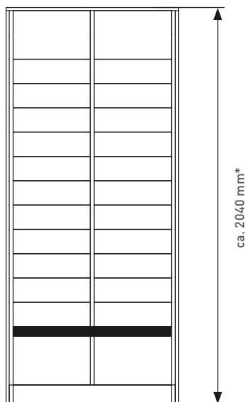
Vista anteriore
